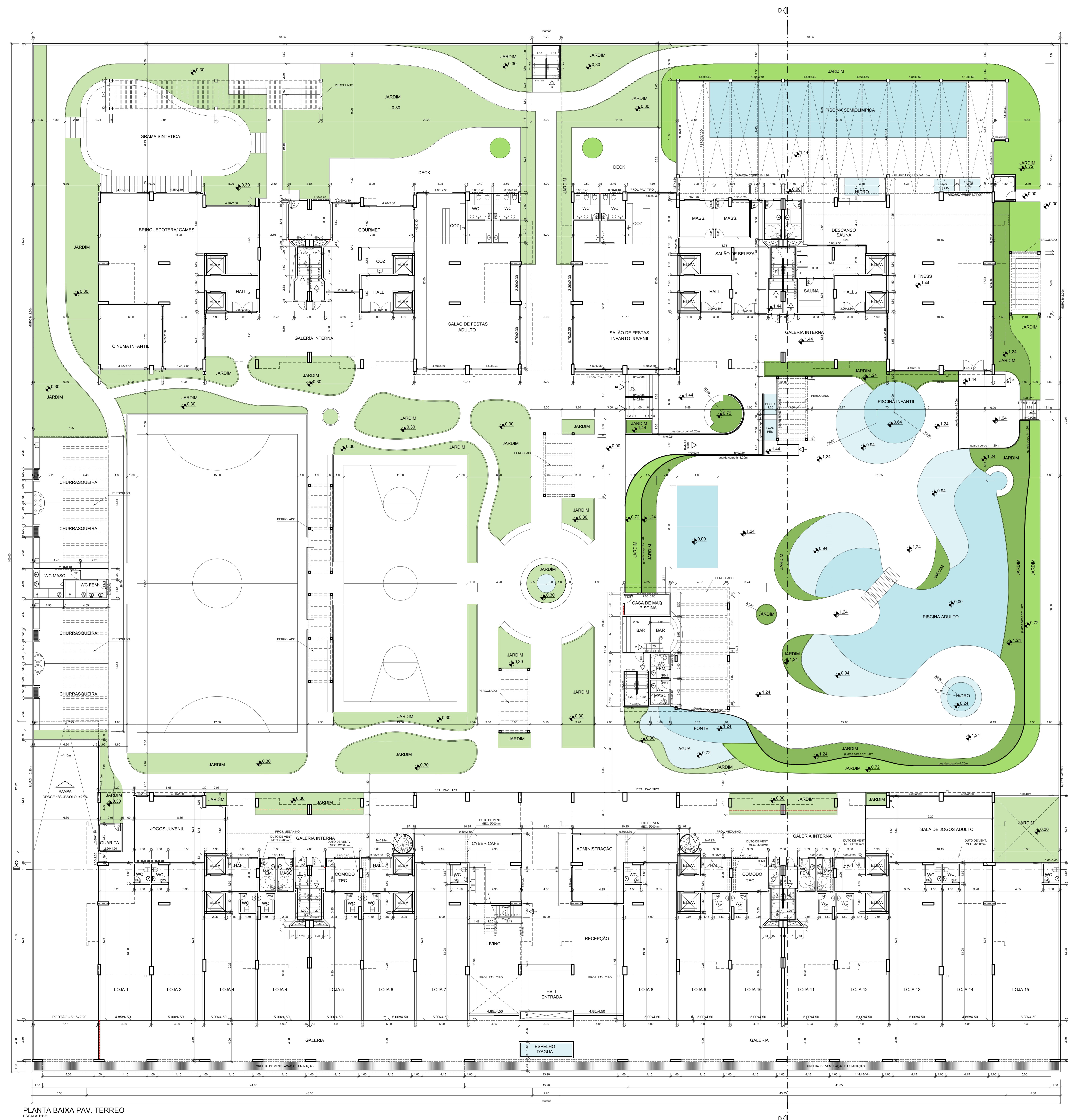
PLANTA BAIXA PAV. TERREO
